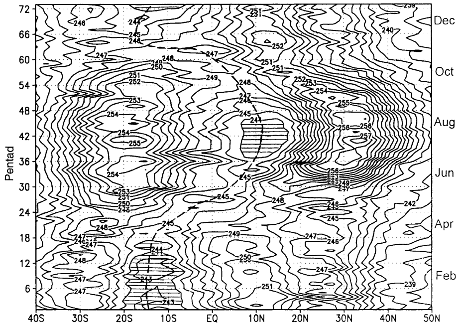
(a) BT, 40-50E
