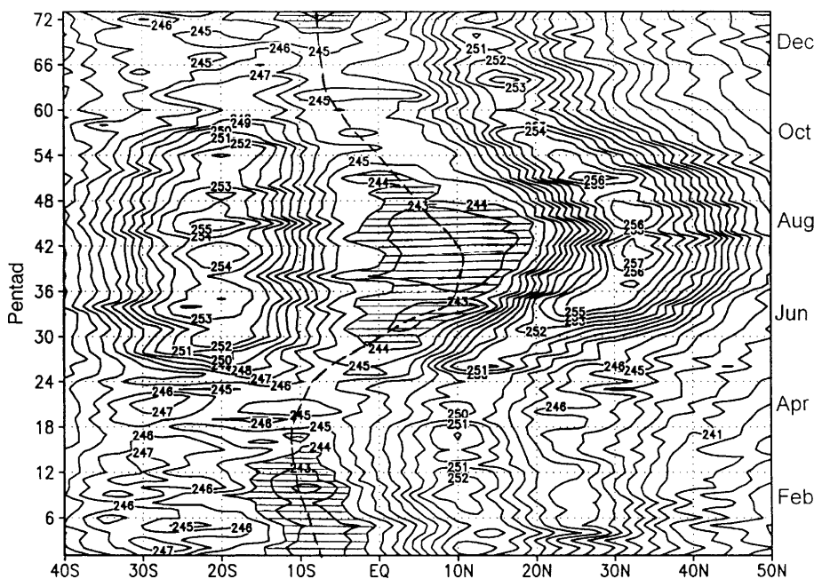
(b) BT, 50-60E
