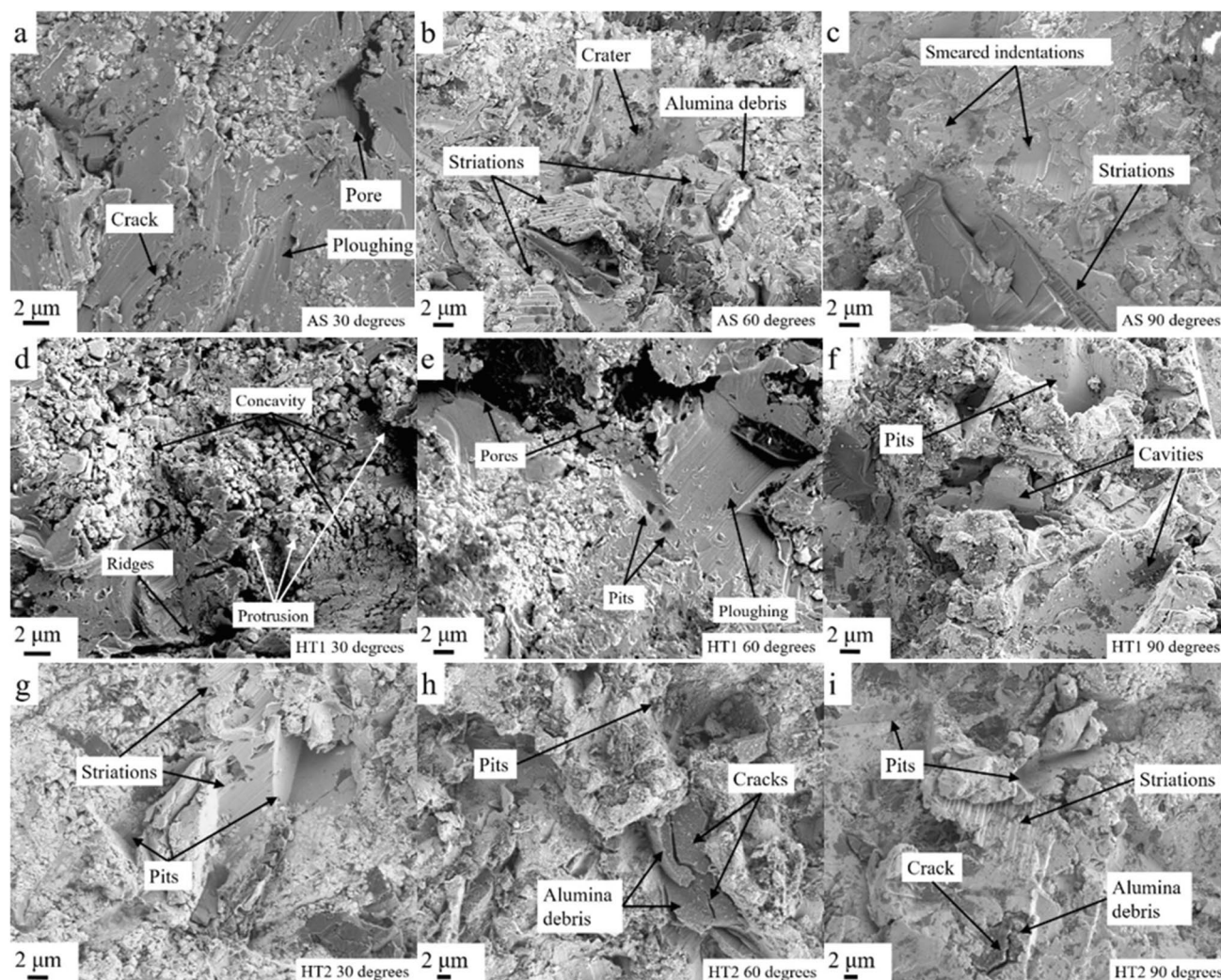
Fig. 10 SEM images of the erosion areas of the WC/Ni coatings: a AS—30°, b AS—60°, c AS—90°, d HT1—30°, e HT1—60°, f HT1—90°, g HT2—30°, h HT2—60°, i HT2—90°
