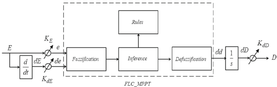
Fig. 4 Bloc diagram of a FLC_MPPT
