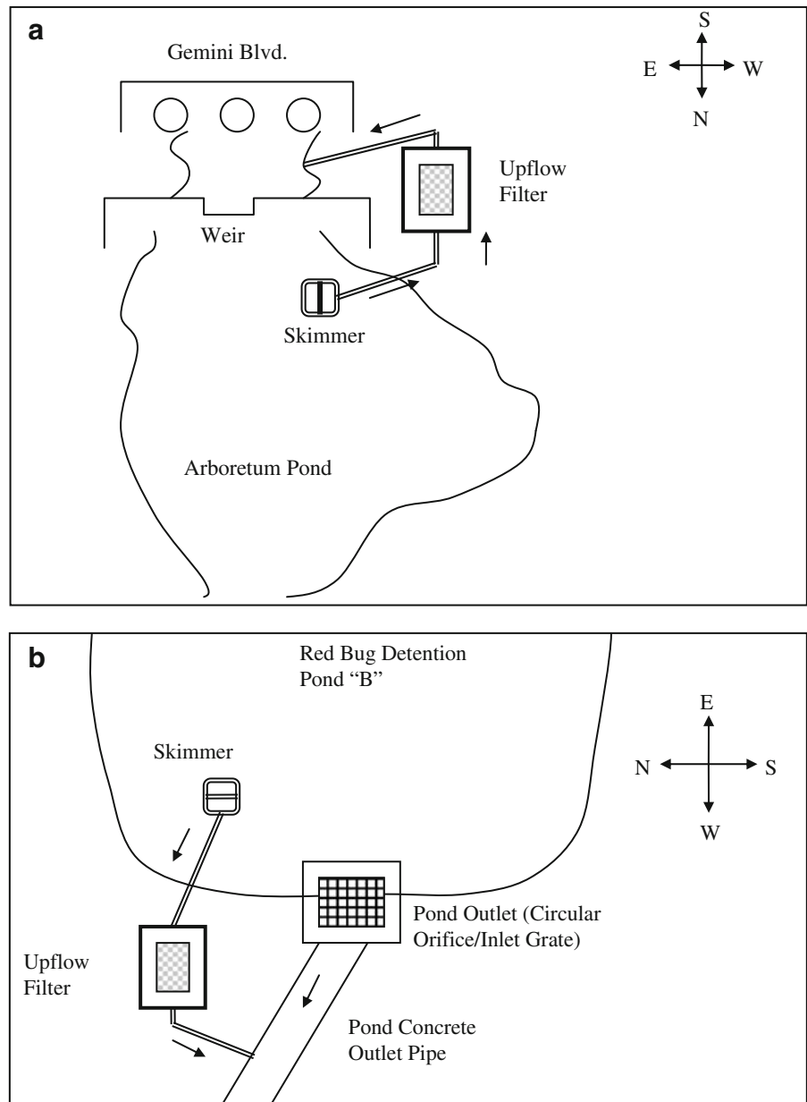
Fig. 3 a Plan view of the Arboretum pond at UCF (N. T.S.), b plan view of Red Bug Pond B in Seminole County (N.T.S.)
