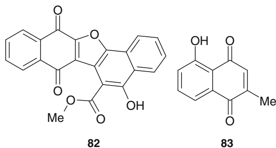
Fig. 4 Quinones
