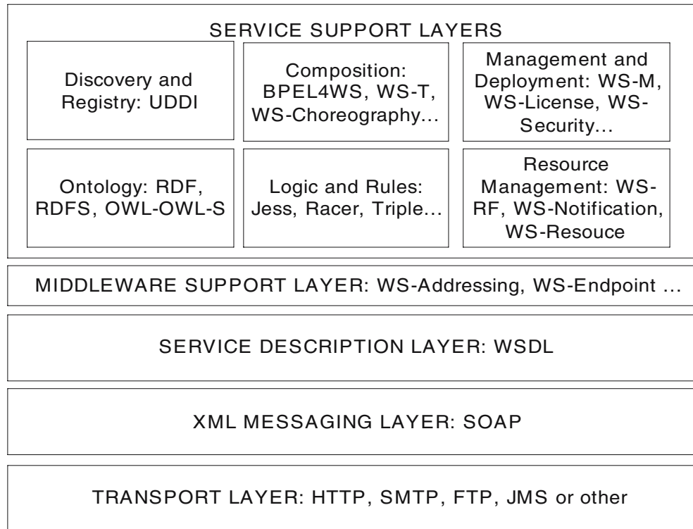
Fig. 1 Web service technologies
