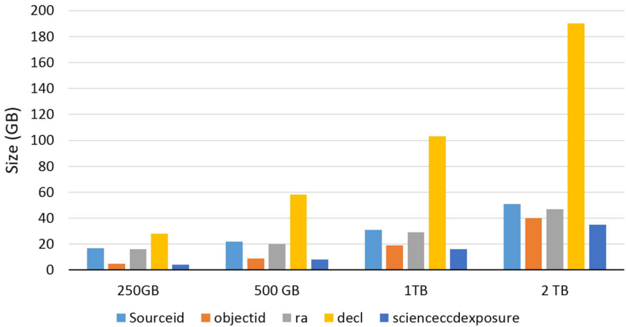
Fig. 4 Hive: index size
