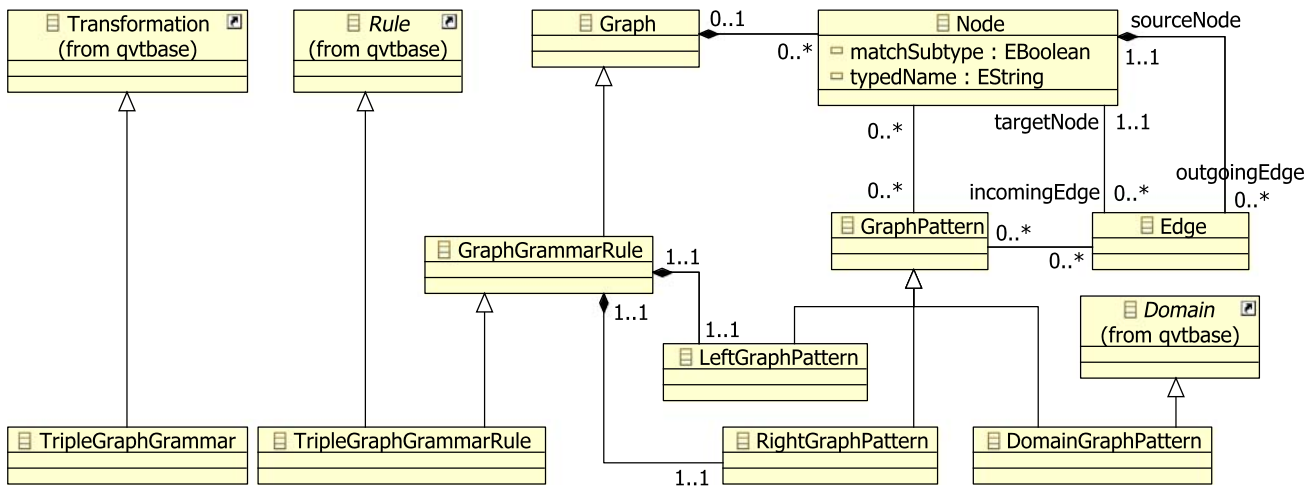
Fig. 15 The TGG meta-model
