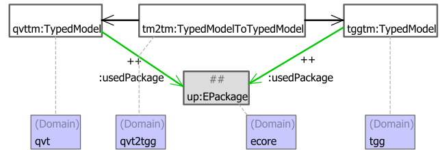
Fig. 19 Rule: UsedPackageToUsedPackage
