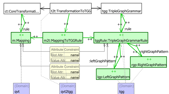
Fig. 17 Rule: MappingToTGGRule
