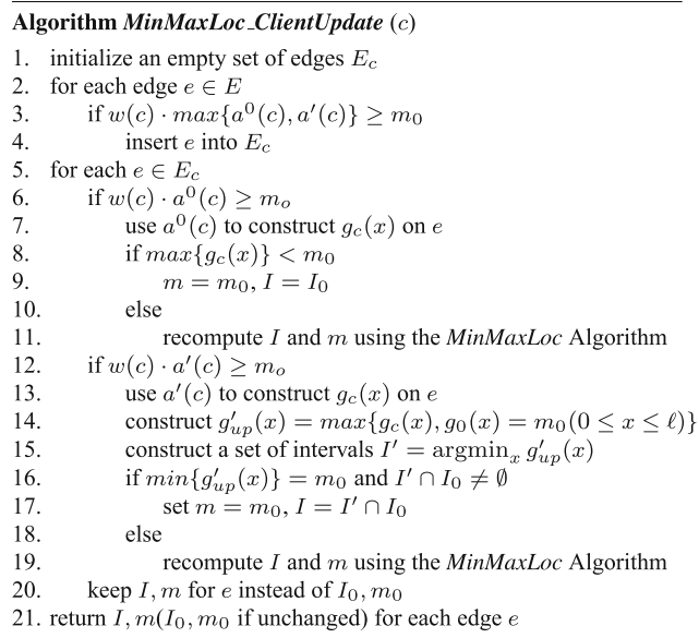
Fig. 15 The MinMaxLoc_ClientUpdate Algorithm
