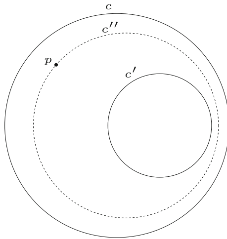
Fig. 32 An illustration of Lemma 5.5
