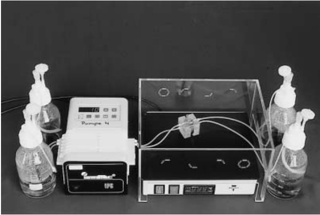
Fig. 1 MINUTH Perfusion Culture Container (MINUCELLS und MINUTISSUE Vertriebs-GmbH, Bad Abbach, Germany)
