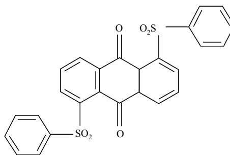
Bis-1,5-(benzenesulfonyl)-9,10-anthraquinone (AQ2)
