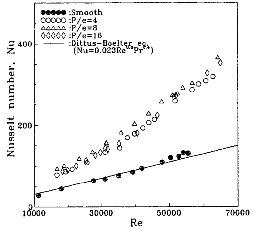
Fig. 6 Nusselt number
