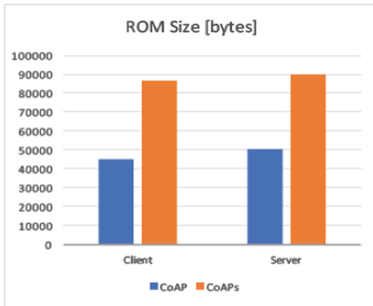
Fig. 11. ROM footprint
