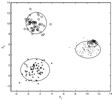
Fig. 7. BIC.
