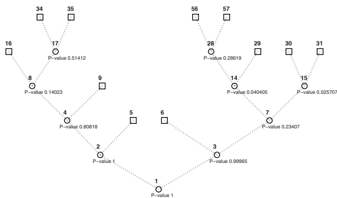
Fig. 1. Posterior prediction modelling tree.
