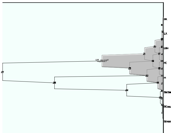
Fig. 1. Pyramid.
