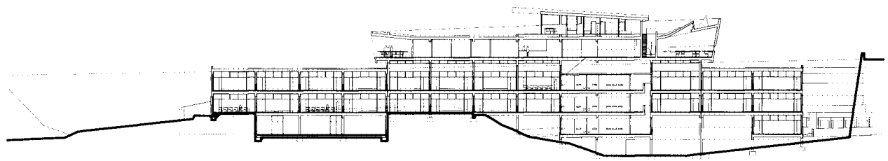
Longitudinal section
