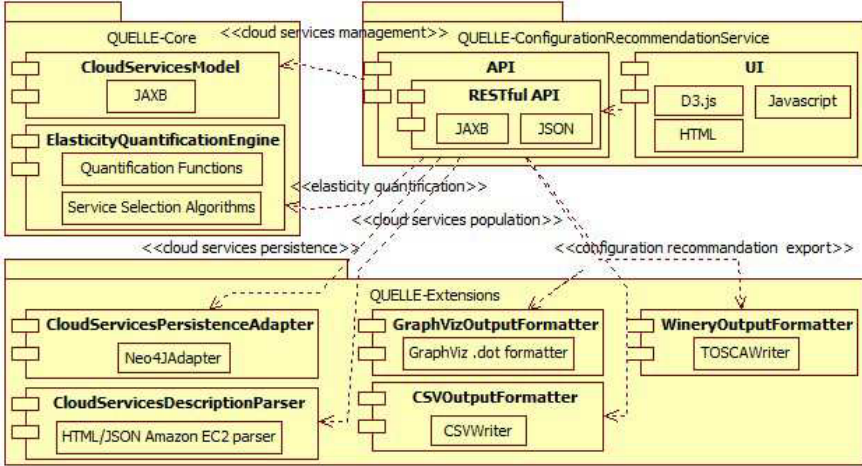
Fig. 4. QUELLE framework
