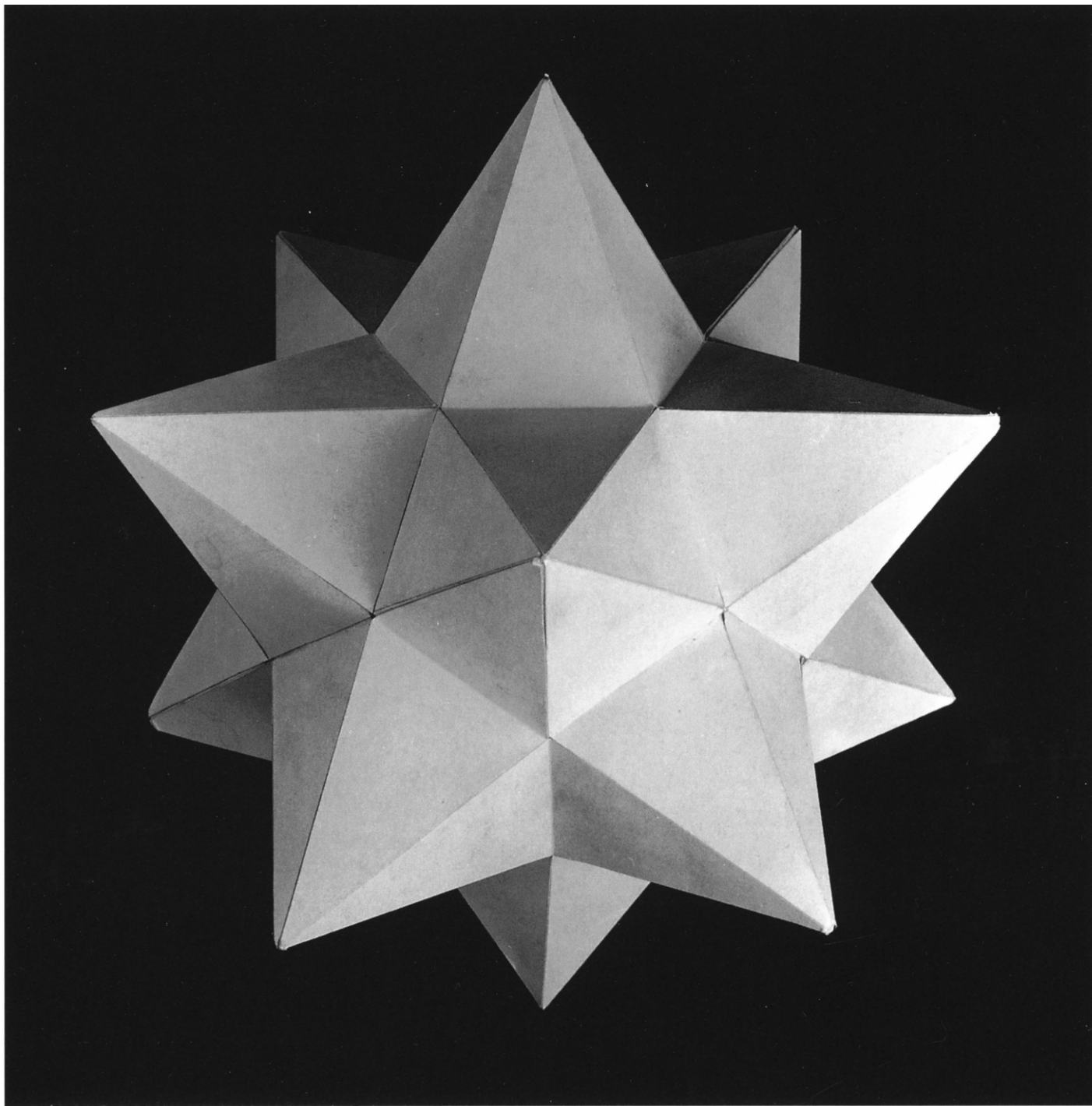
103 Zwölfeckiges Sternzwölfflach (kleines Sterndodekaeder)
