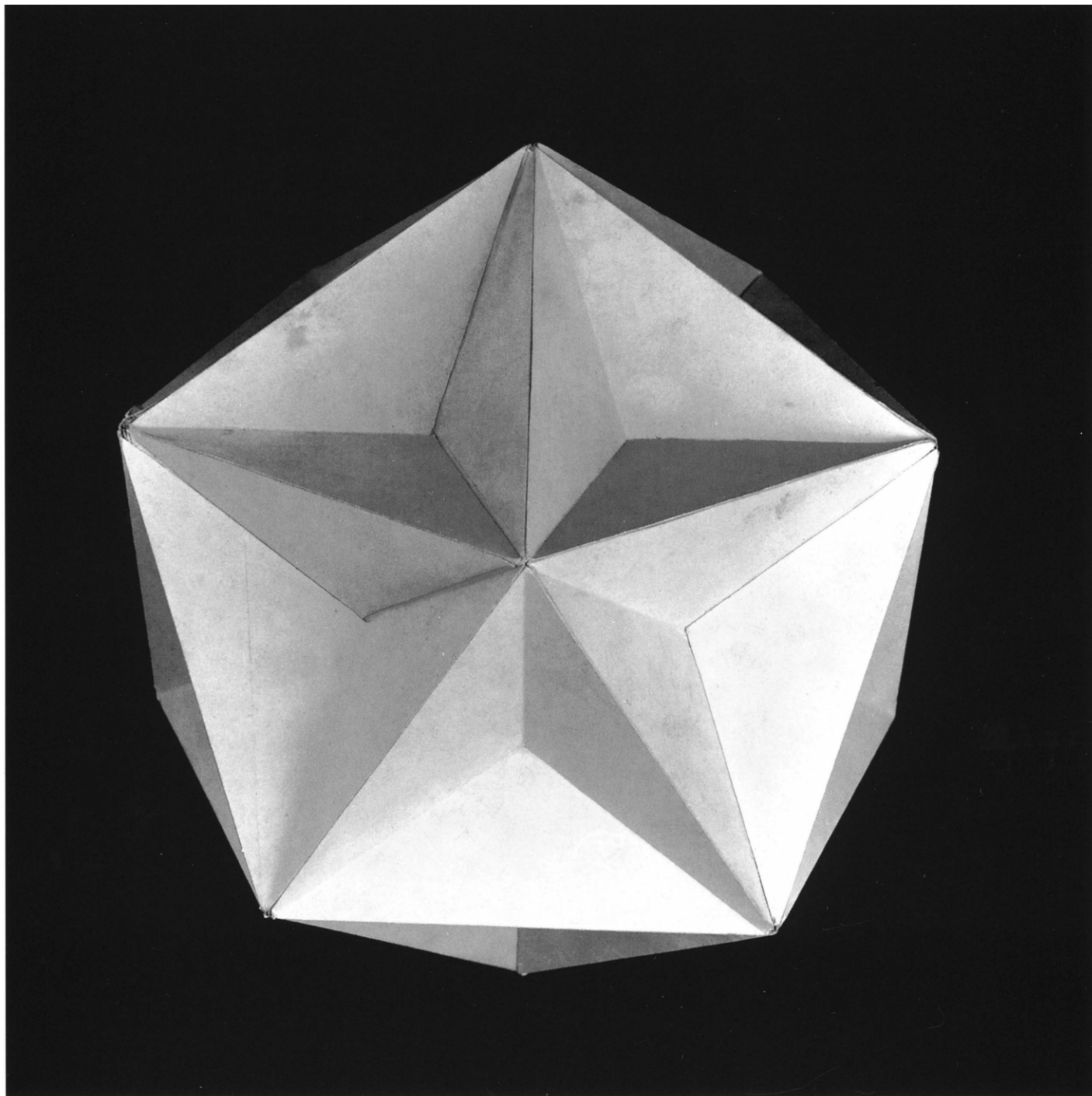
105 Sterneckiges Zwölfflach (großes Dodekaeder)
