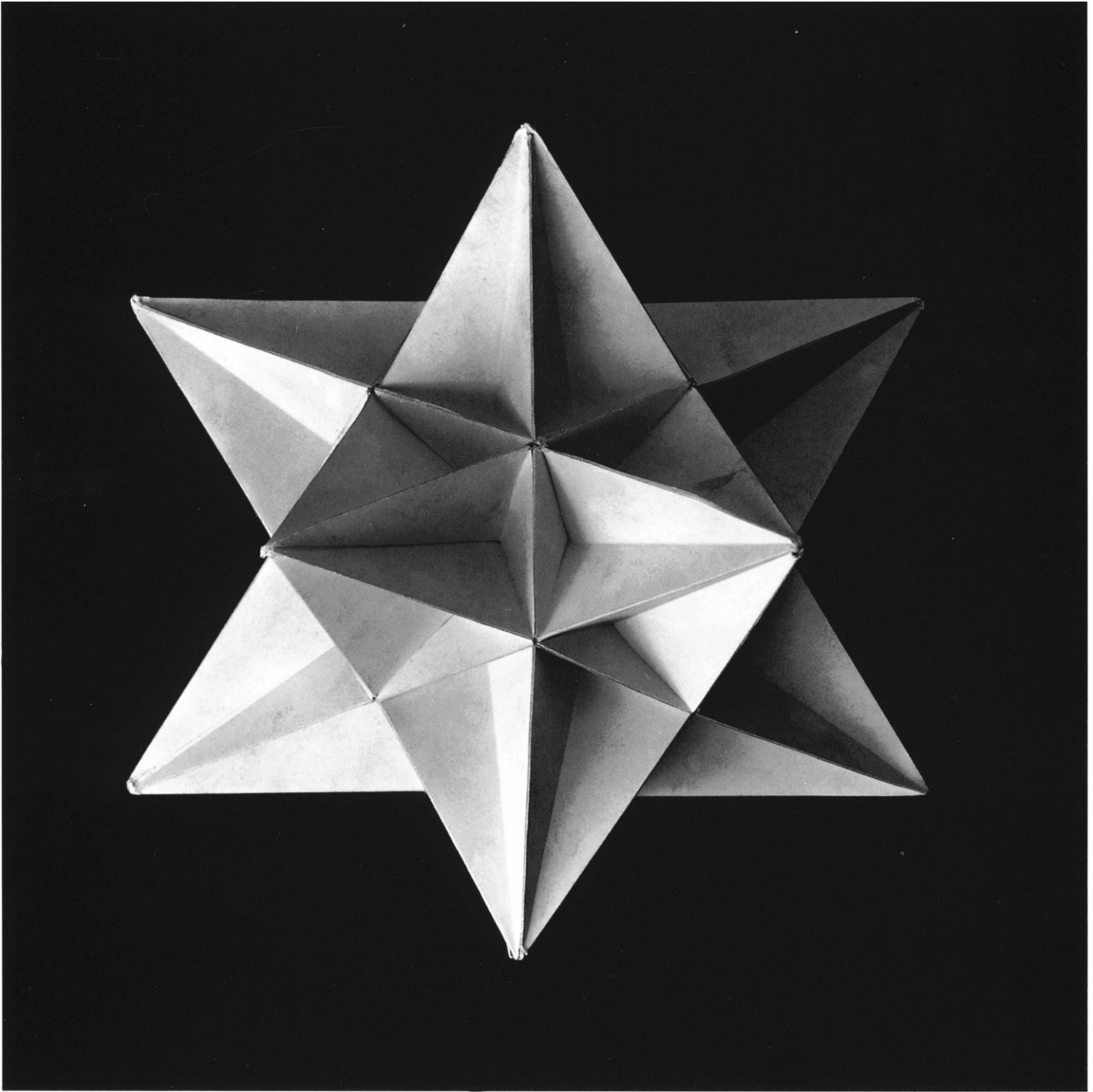
106 Sterneckiges Zwanzigflach (großes Ikosaeder)
