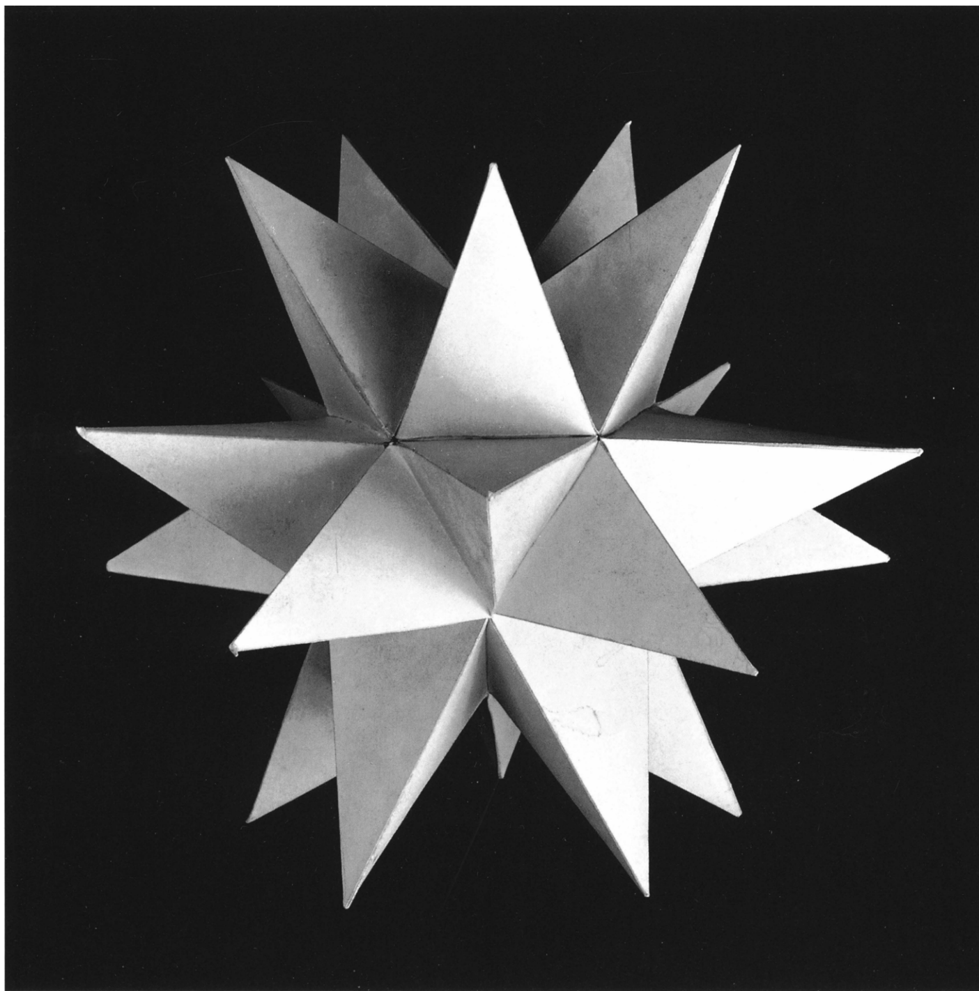
104 Zwanzigeckiges Sternzwölfflach (großes Sterndodekaeder) Great stellated dodecahedron
