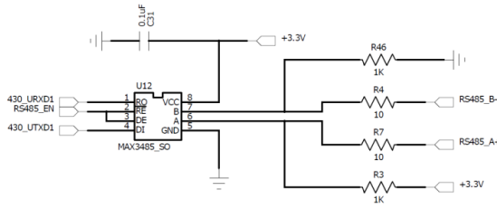
Fig. 6. Communication module
