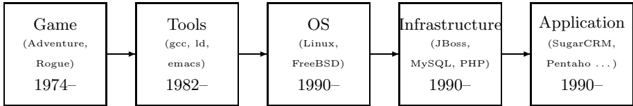
Fig. 1. Augustin’s 5 generation-view
