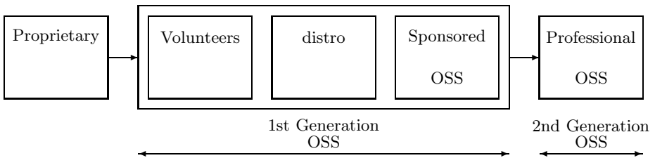
Fig. 2. Watson’s 2 generation-view
