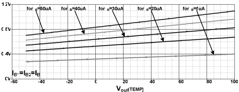
Fig. 7. PTAT reference
