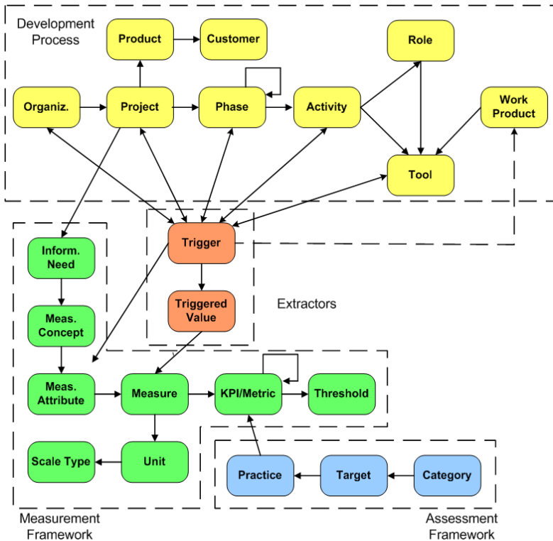
Fig. 3. The Spago4Q meta-model [5]
