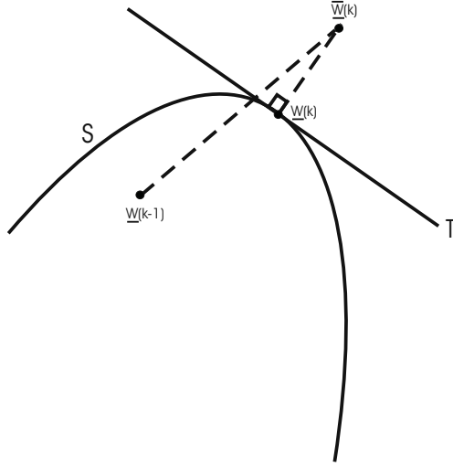
Fig. 7 Discrete Time Parameter Projection
