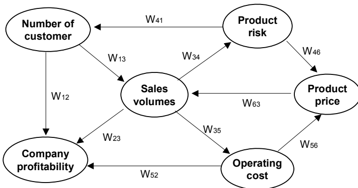
Fig. 1 Simple FCM
