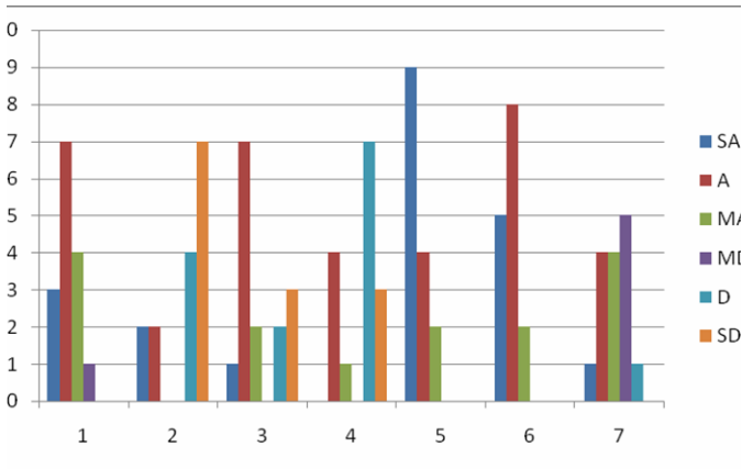
Fig. 3. Questionnaire results
