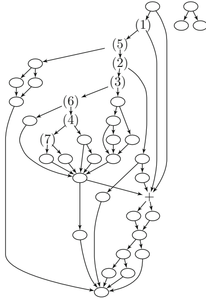
Fig. 7. CFG for sub_60118
