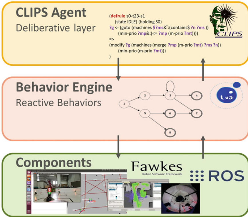
Abbildung 3 Hybride 3-Layer Architektur für die Robocup Logistics League, Team Carolitics Aachen
