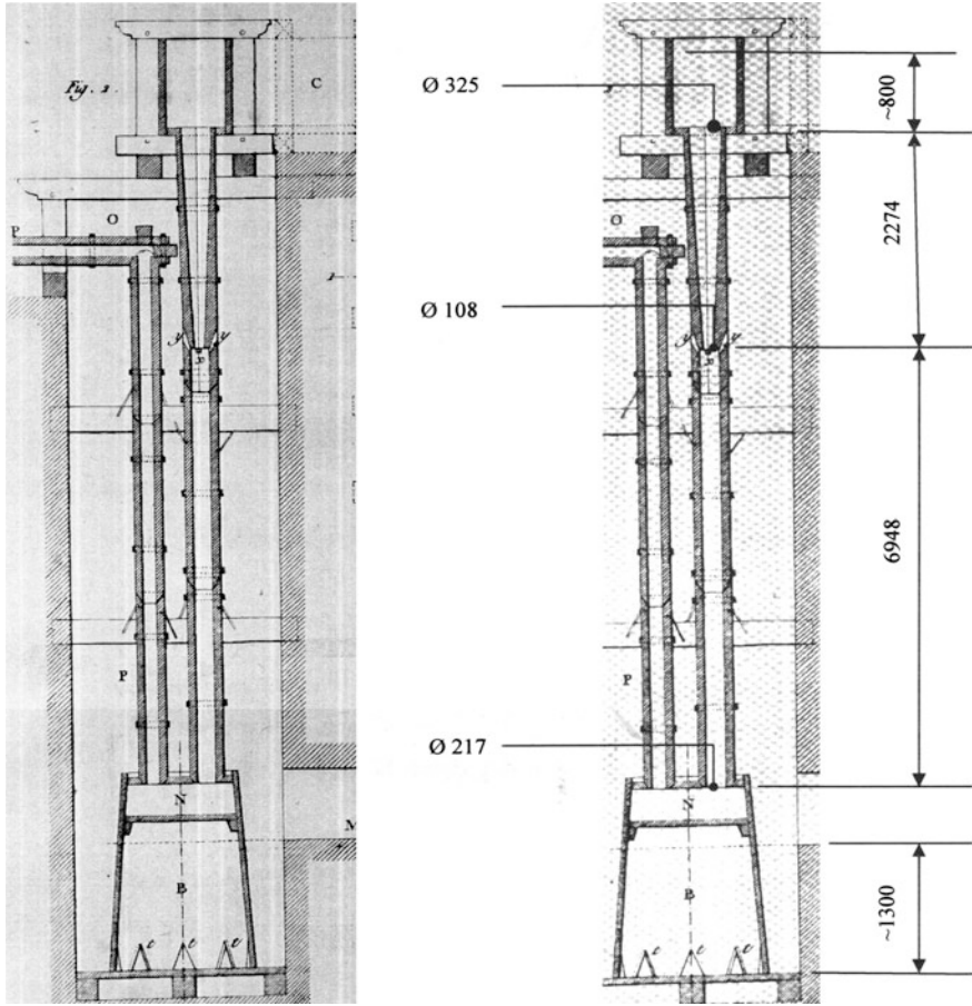
Fig. 15 Detail of the water bellows illustrating the paper “Expériences faites sur les trompes de la Fonderie de Poullaouen” [Beauvier, Gallois]. Dimensions are in mm
