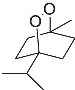
ascaridole
