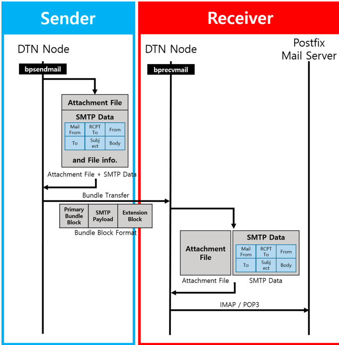
Fig. 5. DTN-SMTP message format & flow
