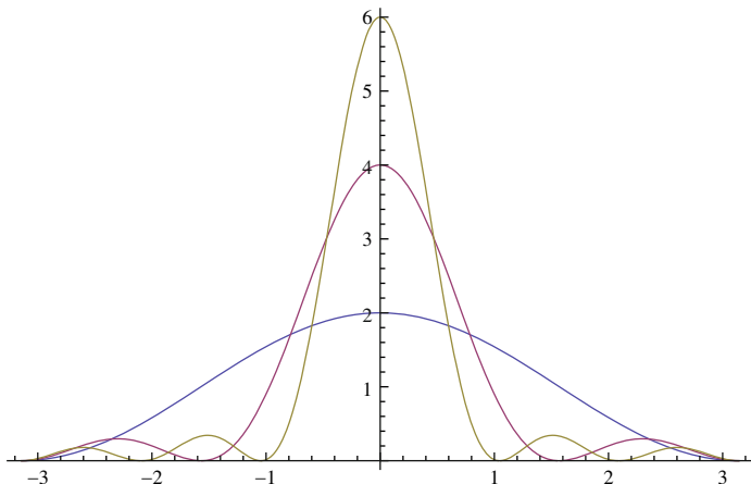
FIGURE 4. Fejer kernel
