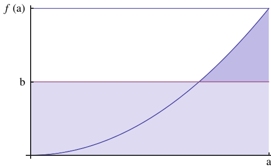
FIGURE 3. Lemma 3.5
