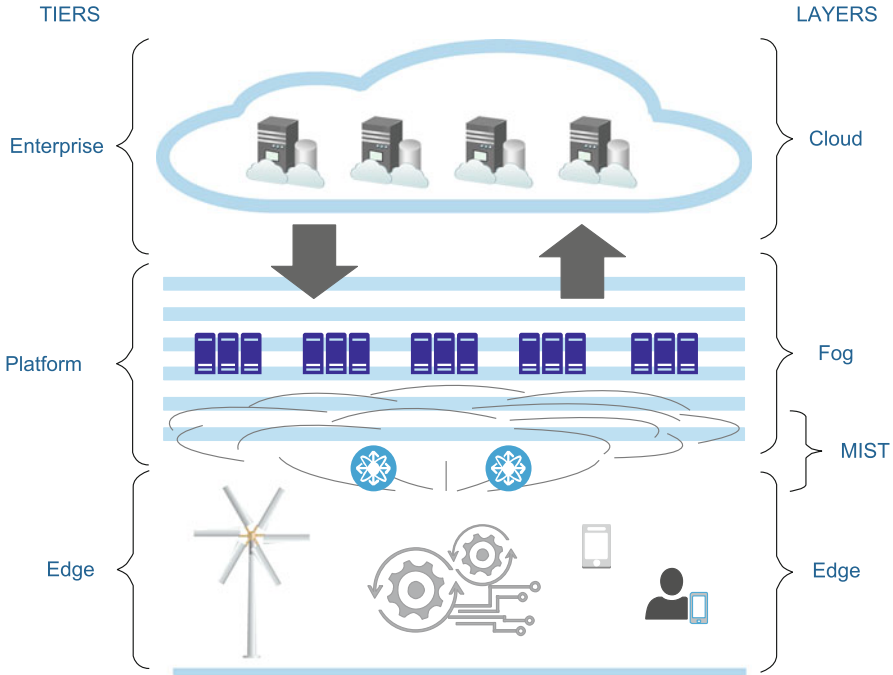
Fig. 1 IIoT Ecosystem
