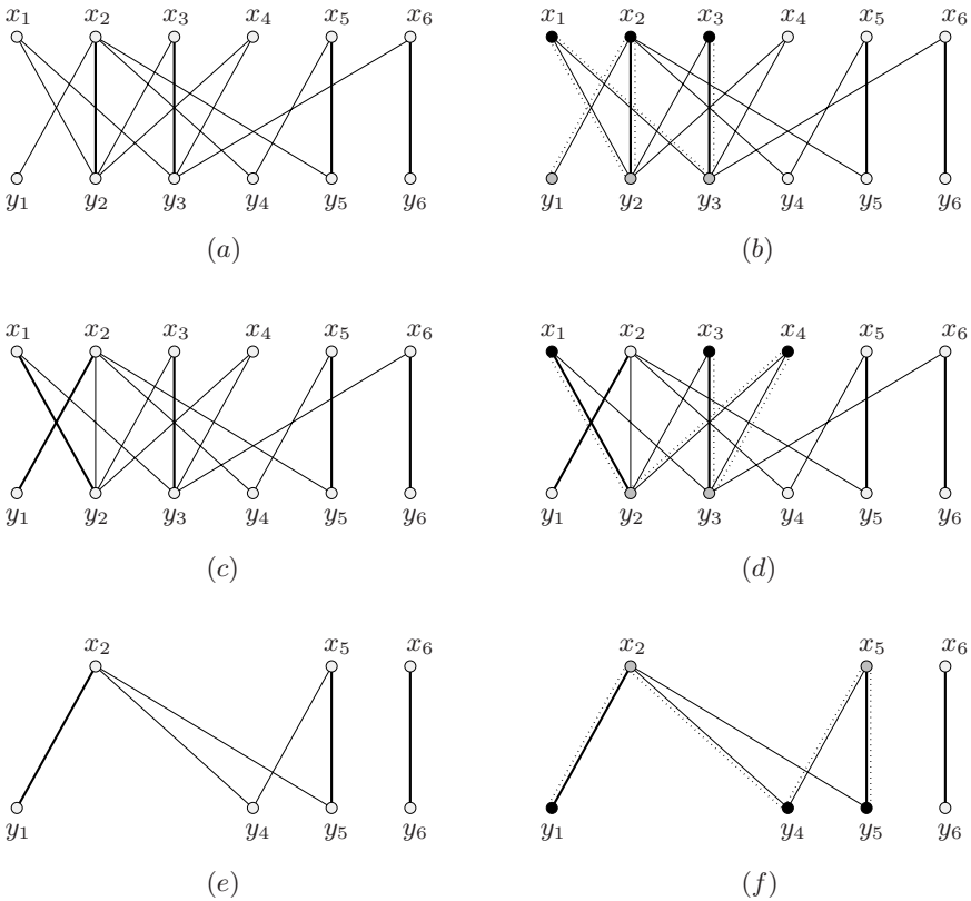
Fig. 16.12. Egerváry’s Algorithm: finding a maximum matching in a bipartite graph
