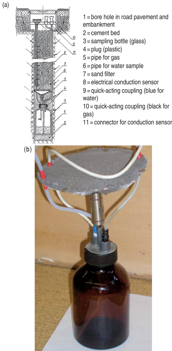
Fig. 7.8 (a) Seeping waters sampler in road embankment (Sytchev, 1988, modified in Jandová, 2006). Reproduced by permission of Centrum Dopravního Výzkumu, v.v.i. (b) Sampling bottle, valve and “area lysimeter” (Jandová, 2006). Reproduced by permission of Centrum Dopravního Výzkumu, v.v.i.
