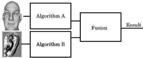
(d) Multi-modal
