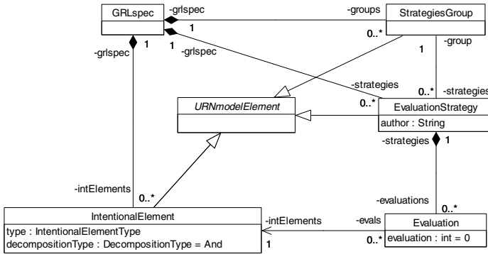
Fig. 9. Evaluation strategies metamodel
