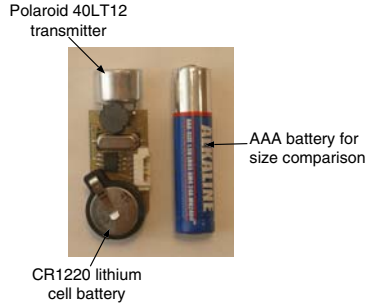
Fig. 1. Ultrasonic Tag
